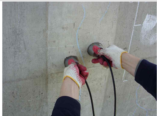
균열깊이 측정현황
